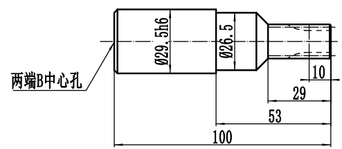
标准“A”型输入轴
